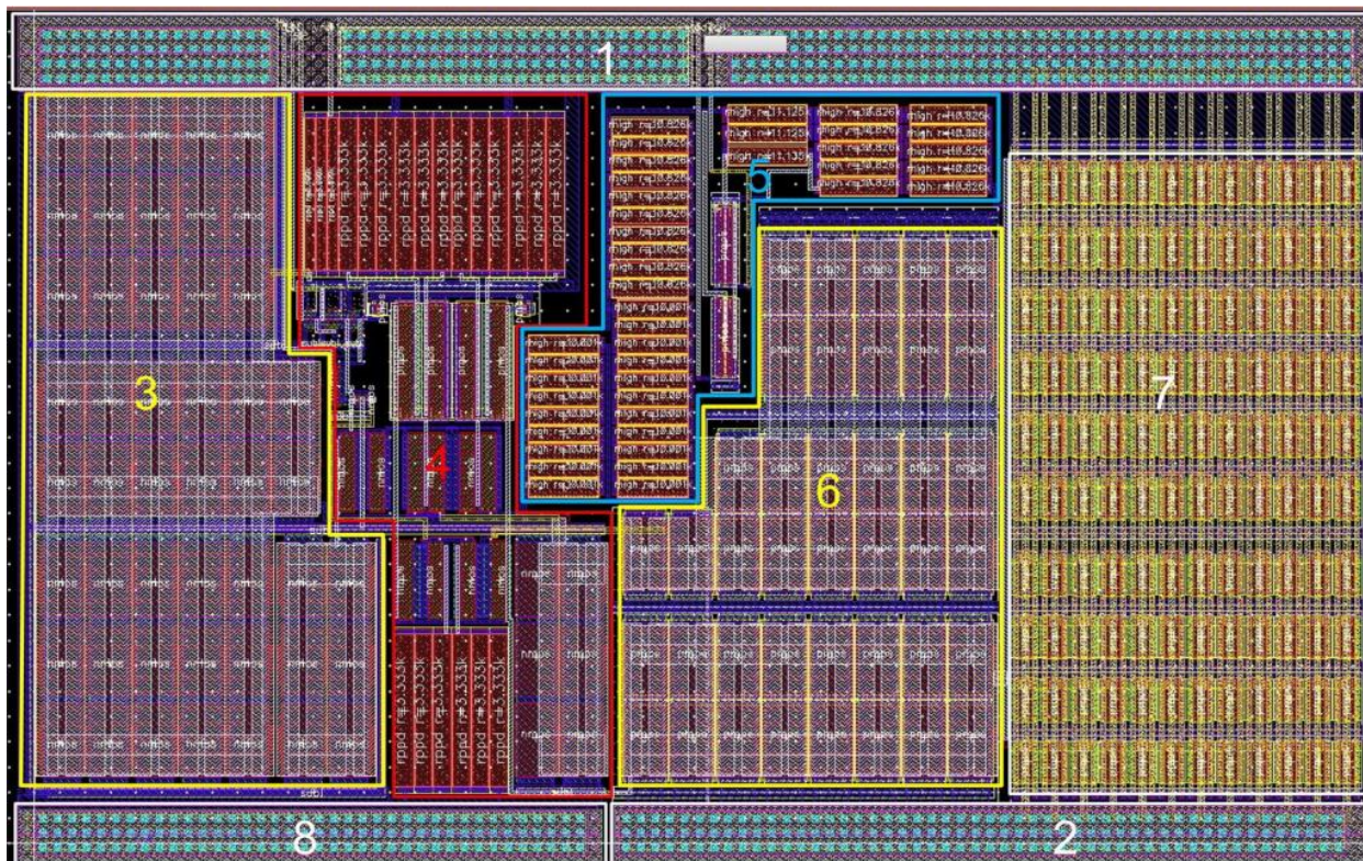
Рисунок 2: Общий вид топологии блока программируемого регулятора напряжения
