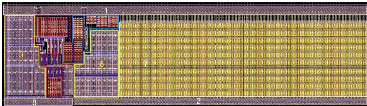
Рисунок 2: Общий вид топологии блока программируемого регулятора напряжения
