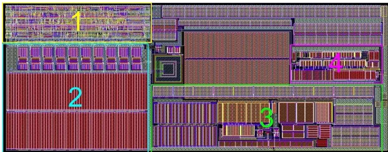
Рисунок 2: Общий вид топологии блока датчика температуры.
