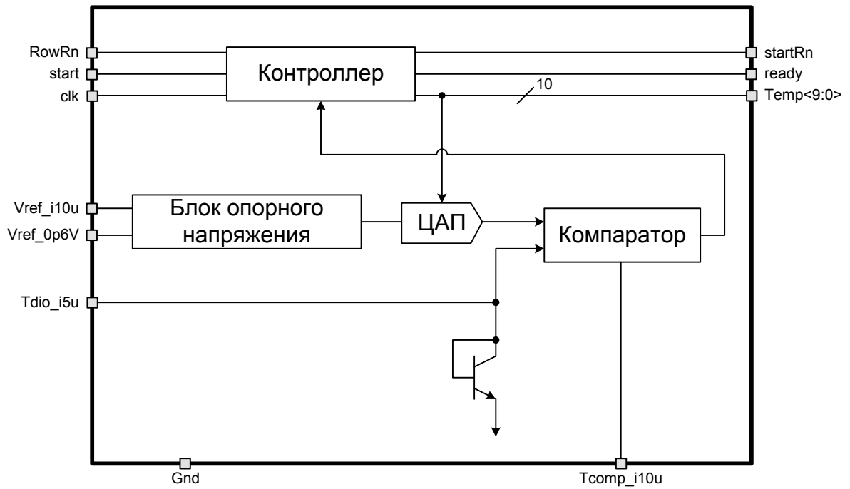
Рисунок 1: Блок-схема датчика температуры.
