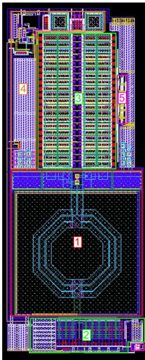
Рисунок 2: Общий вид топологии блока ГУН.
