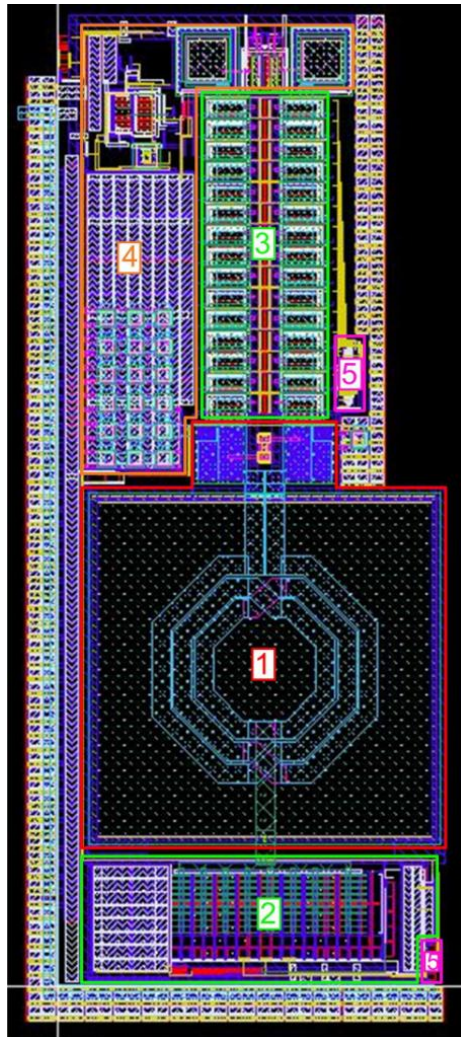
Рисунок 2: Общий вид топологии ГУН.
