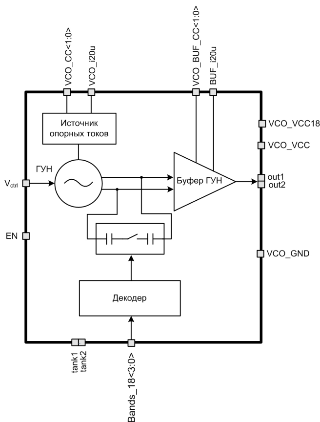
Рисунок 1: Блок-схема ГУН.
