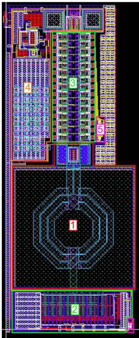
Рисунок 2: Общий вид топологии блока ГУН.
