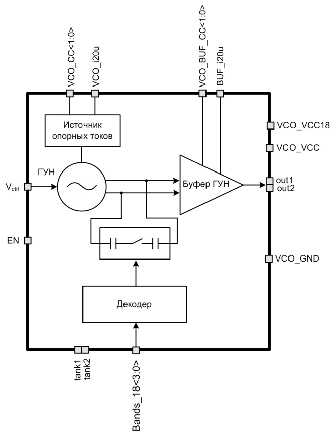
Рисунок 1: Блок-схема ГУН.
