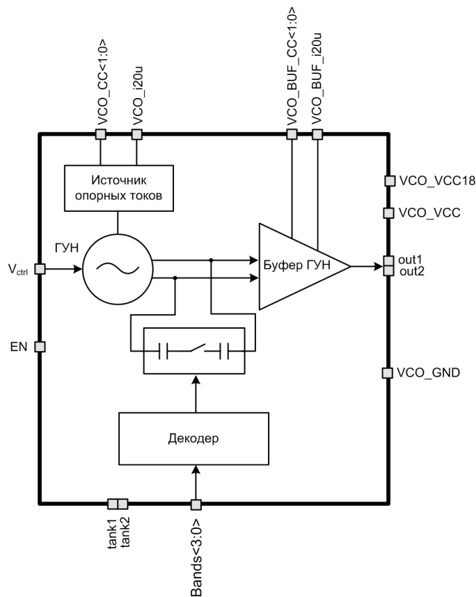
Рисунок 1: Блок-схема ГУН.
