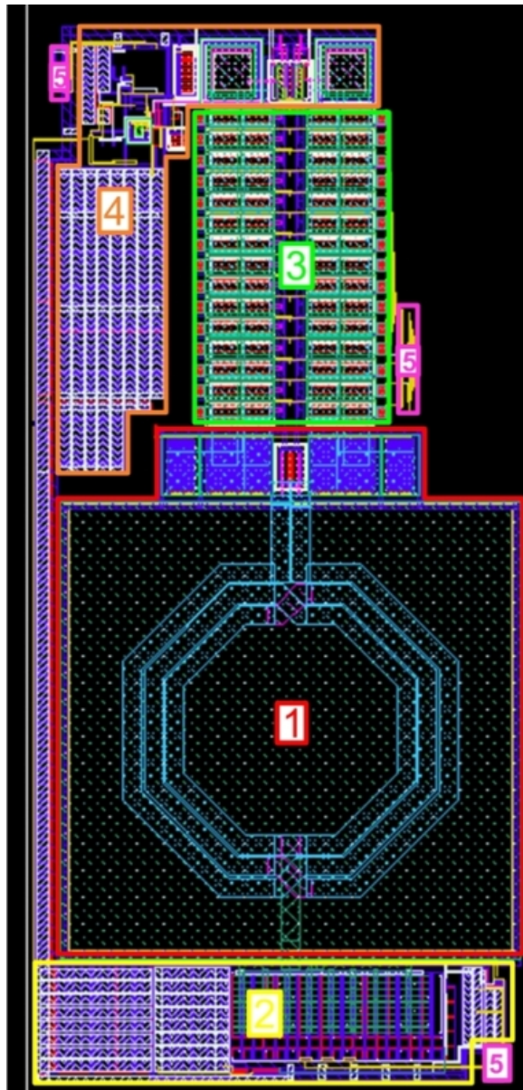
Рисунок 2: Вид топологии блока ГУН.
