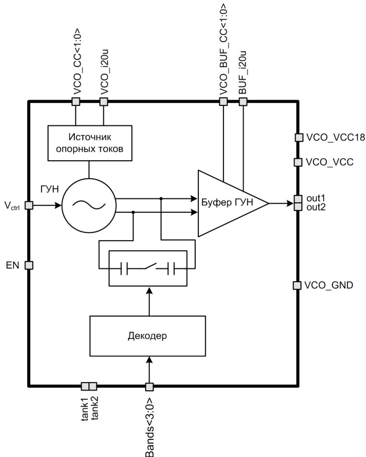
Рисунок 1: Блок-схема ГУН.
